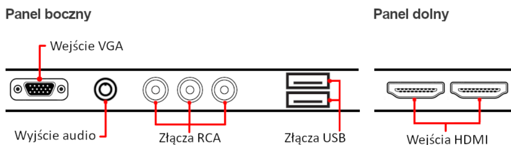
Opis złączy monitora IPOX PX-M43.
